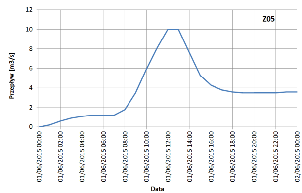
Ryc. 153. Zestawienie hydrogramów przepływu Q_{\max p}=1\% dla Z04 cz.2, Z05 Źródło: opracowanie własne
