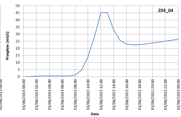
Ryc. 152. Zestawienie hydrogramów przepływu Q_{\max p=1\%} dla Z02, Z03, Z04 cz. 1 Źródło: opracowanie własne
