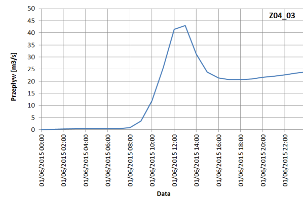
Ryc. 152. Zestawienie hydrogramów przepływu Q_{\max p=1\%} dla Z02, Z03, Z04 cz. 1 Źródło: opracowanie własne
