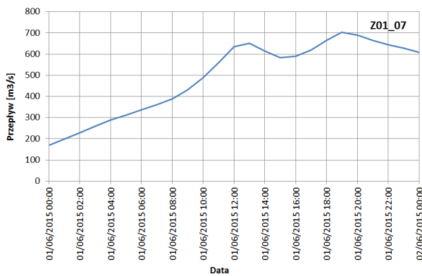
Ryc. 150. Zestawienie hydrogramów przepływu Q_{\max}=1\% dla Z01, cz. 1 Źródło: opracowanie własne
