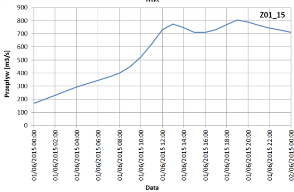
Ryc. 151. Zestawienie hydrogramów przepływu Q_{\max}=1\% dla Z01, cz. 2 Źródło: opracowanie własne
