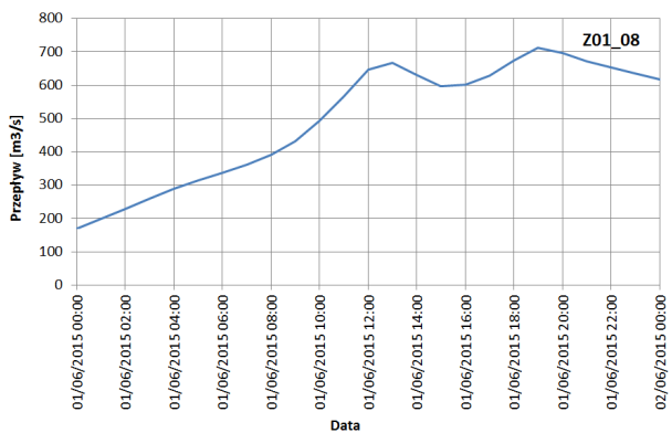
Ryc. 150. Zestawienie hydrogramów przepływu Q_{\max}=1\% dla Z01, cz. 1 Źródło: opracowanie własne
