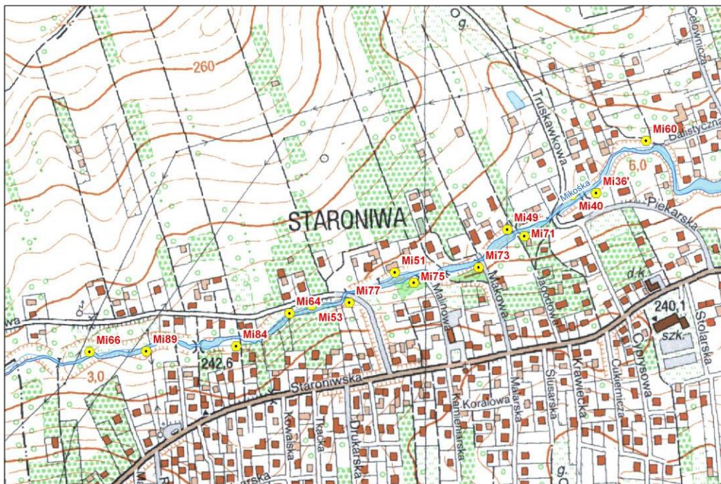
Ryc. 121. Lokalizacja wylotów kanalizacji deszczowej do potoku Mikoška - cz. 1
