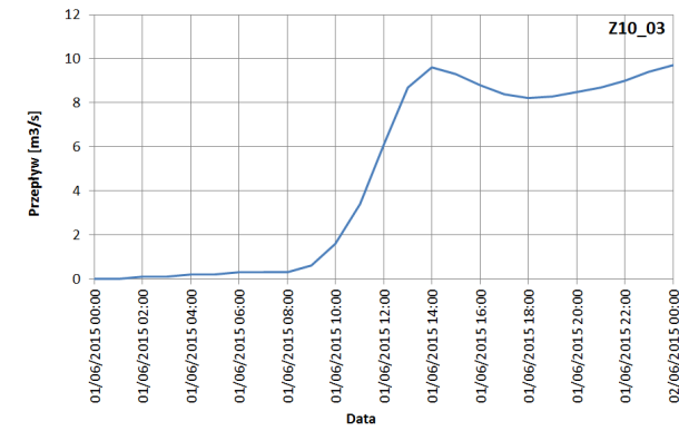
Ryc. 154. Zestawienie hydrogramów przepływu Q_{\max p}=1\% dla Z06, Z07, Z08, Z09, Z10 cz. 1 Źródło: opracowanie własne
