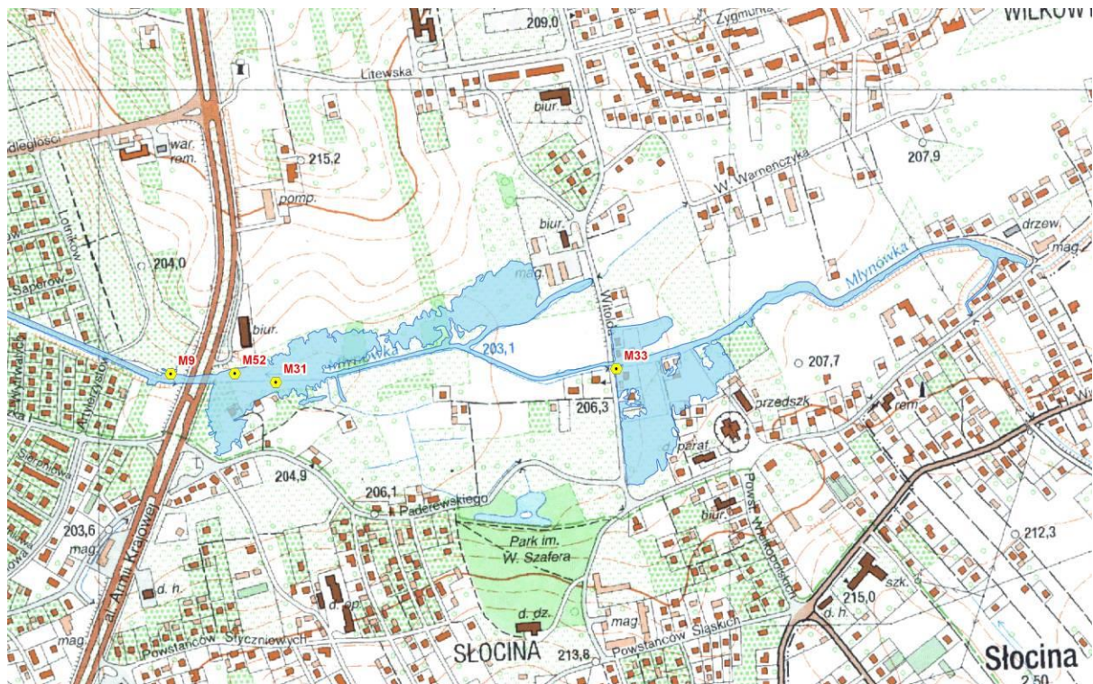
Ryc. 129. Lokalizacja wylotów kanalizacji deszczowej do potoku Młynówka
