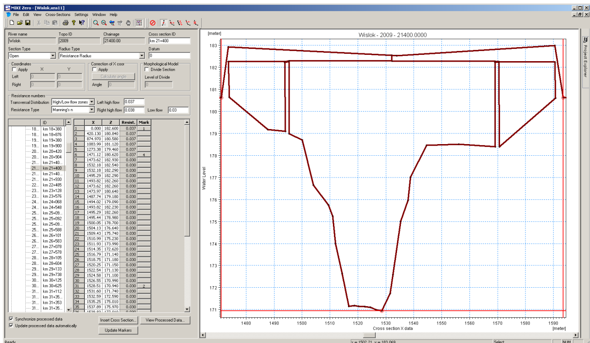
Ryc. 114. Most na Wiśtoku w Budach Łańcuckich wprowadzony do modelu hydraulicznego Źródło: opracowanie własne
