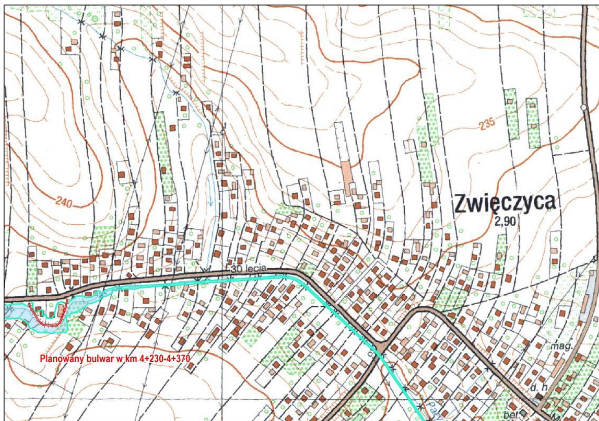
Ryc. 125. Lokalizacja planowanego bulwaru na lewym brzegu Paryji Źródło: opracowanie własne na podstawie mapy topograficznej
