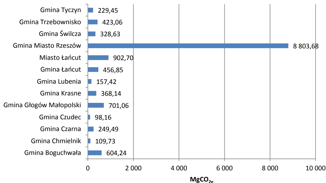
Rysunek 22. Bilans emisji CO 2e w 2010 roku w sektorze oświetlenia publicznego Rzeszowskiego Obszaru Funkcjonalnego 76
