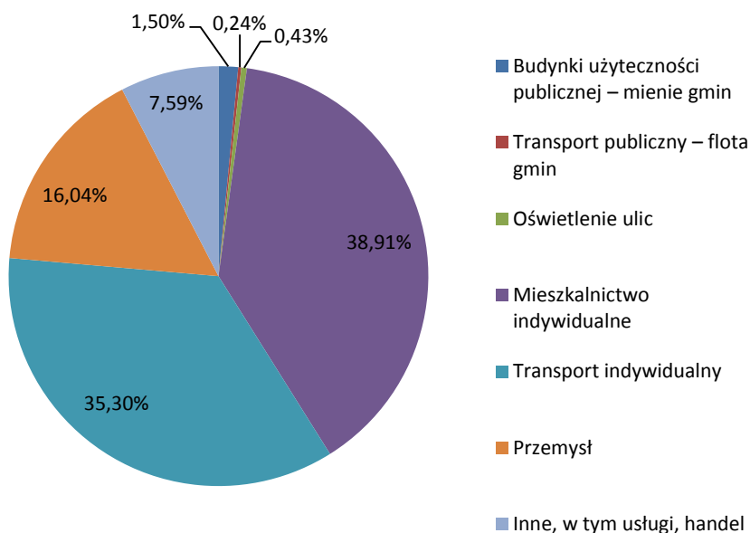
Rysunek 39. Procentowy udział sektorów w ogólnym bilansie emisji CO 2e w gminie Głogów Małopolski 107
