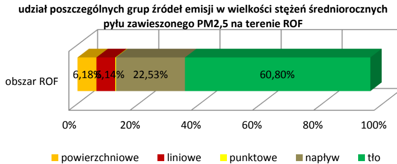
Rysunek 68. Udział poszczególnych źródeł emisji w wielkości stężeń średniorocznych pyłu zawieszonego PM2,5 na terenie ROF w 2013 roku 287
