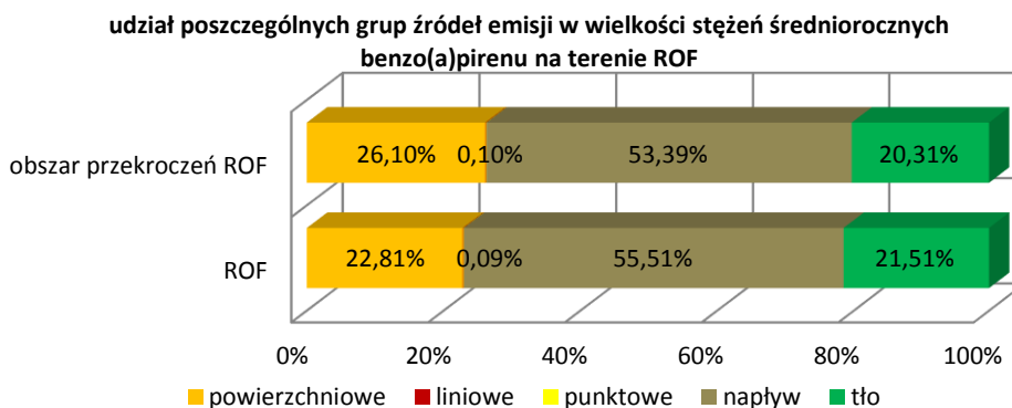
Rysunek 69. Udział poszczególnych źródeł emisji w wielkości stężeń średniorocznych benzo(a)pirenu na terenie ROF w 2013 roku 289
