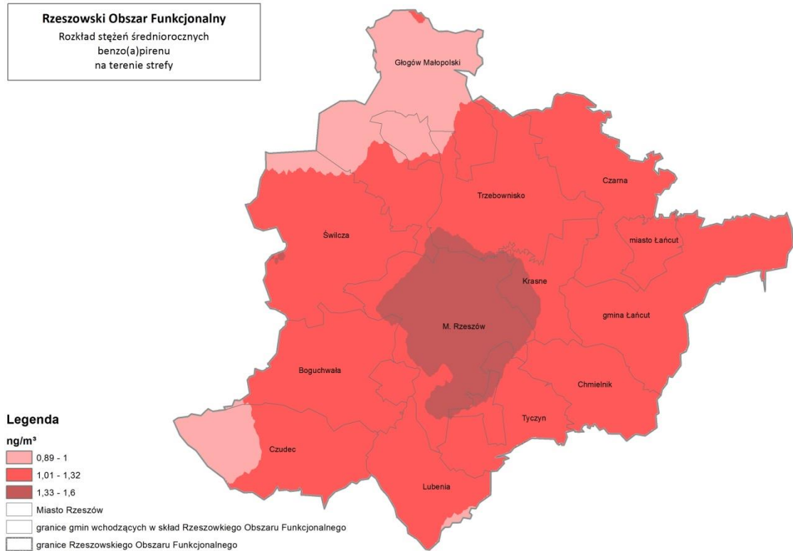
Rysunek 71. Rozkład stężeń średniorocznych benzo(a)pirenu w Rzeszowskim Obszarze Funkcjonalnym w roku bazowym 2013 292
