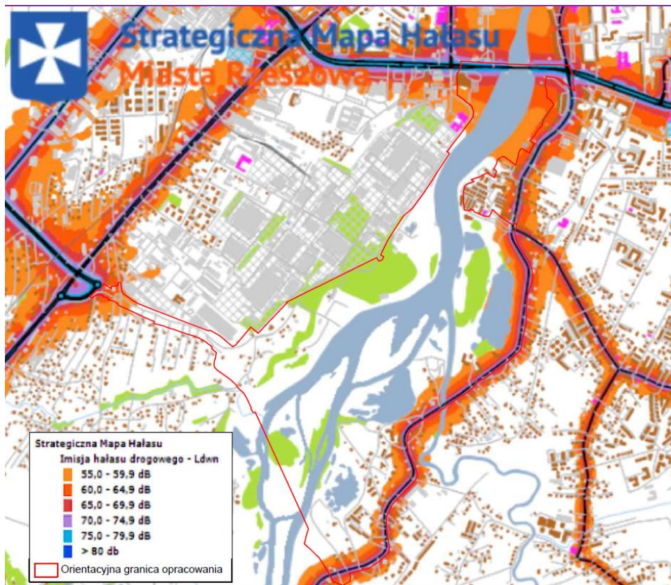
Rys. Strategiczna mapa hałasu drogowego Ldwn w granicy opracowania przyjętej uchwałą
