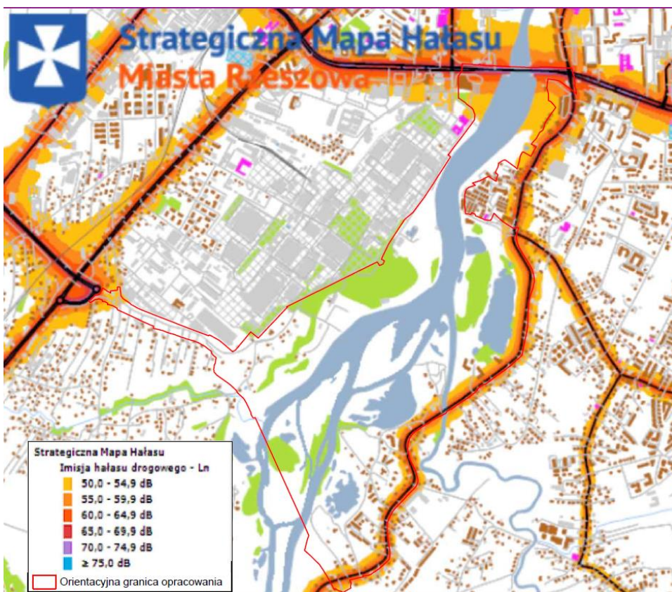
Rys. Strategiczna mapa hałasu kolejowego Ln w granicy opracowania przyjętej uchwałą
