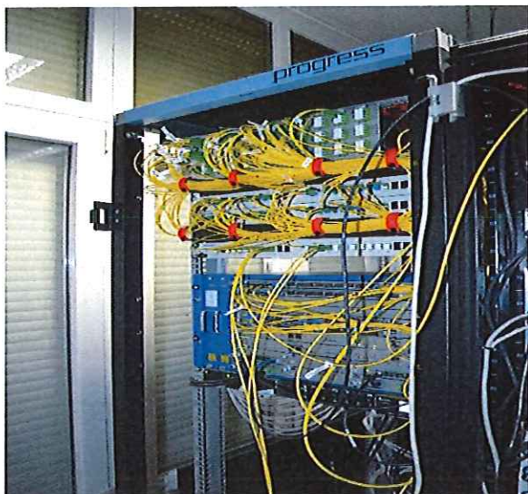
PTITS -łącznica światłowodowa w DATA center, światłowód
